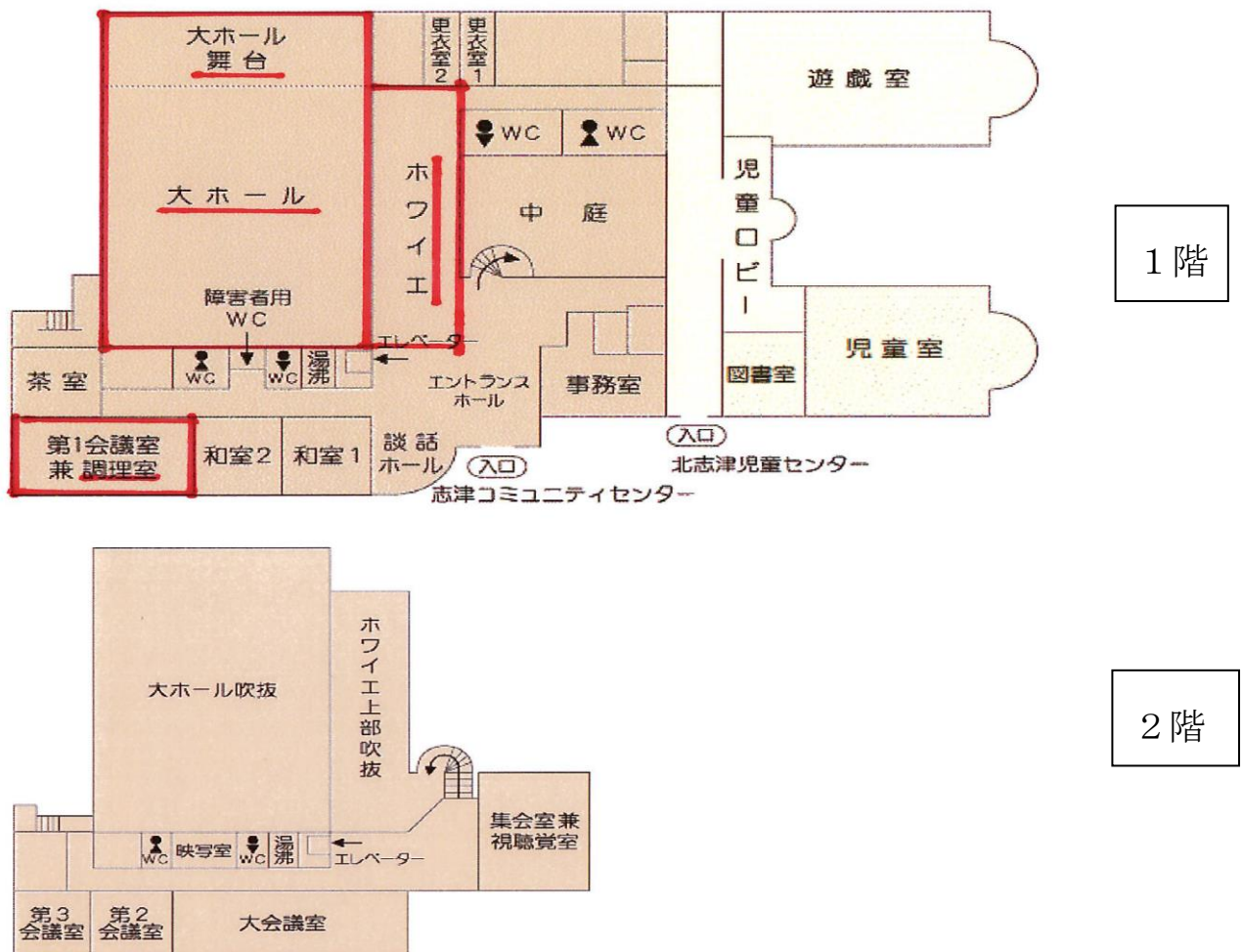
志津コミュニティーセンター施設配置図
